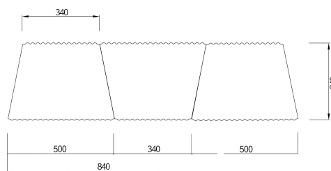
마감(캡) 조립도
